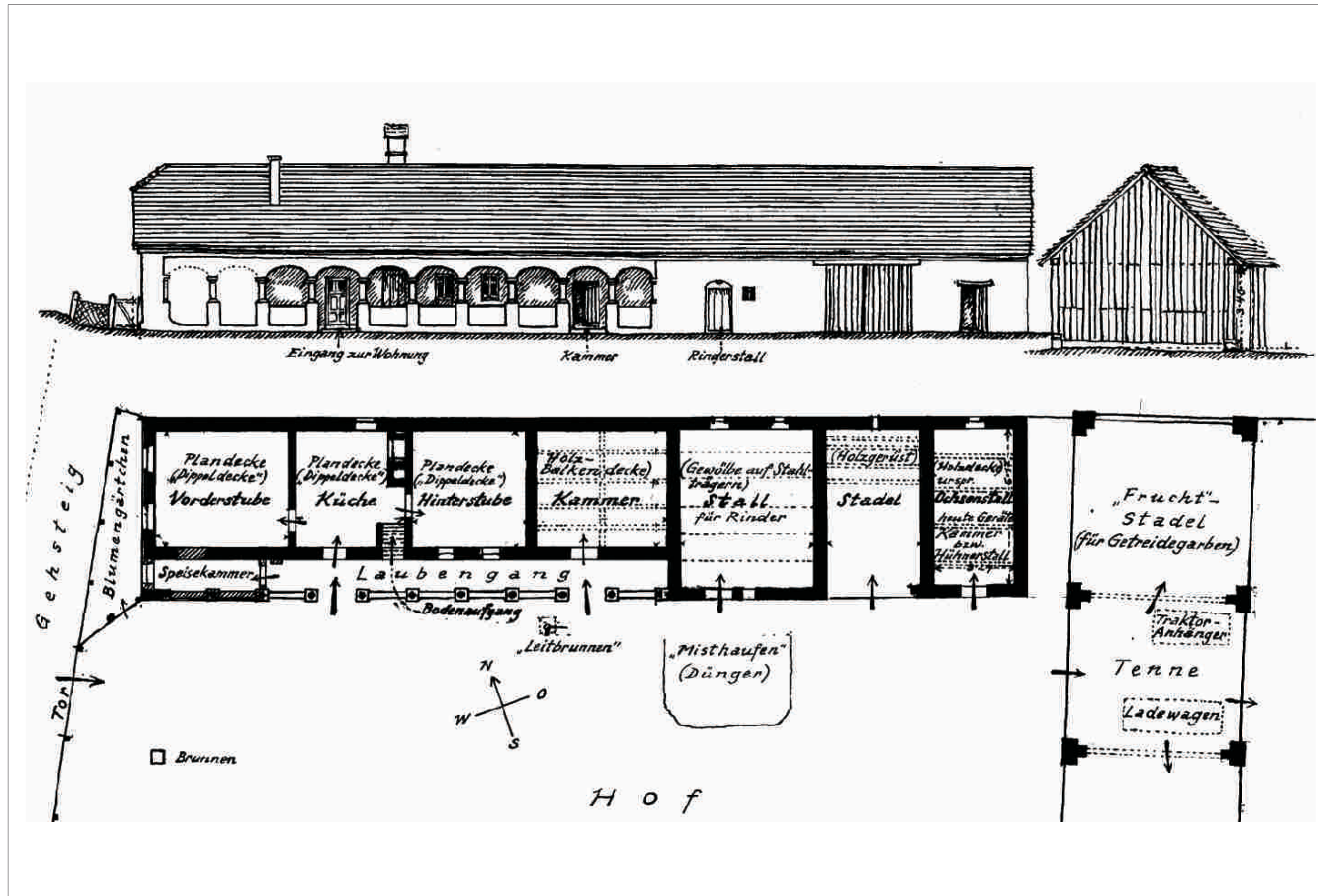
typisches Beispiel eines traditionellen Streckhofs - Grund- und Aufriss (nach Franz Simon 1990)
